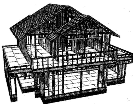
2X4CAD(XF24)の全体パース図
