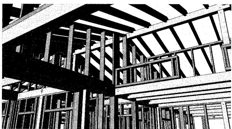
パネル化は金物工法+2×4の「いいとこ取り」で (SIパネルCAD)
