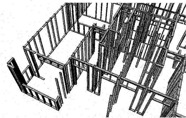
パネル枠組(堅枠パース図)
