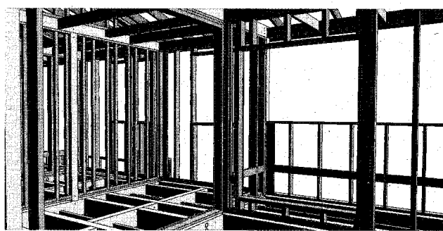
軸組パネル工法は外壁だけでなく、内部造作まで (SIパネルCAD)
