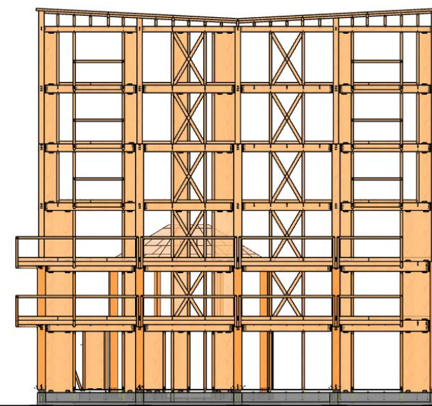
北立面図
