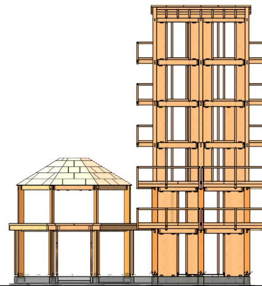
東立面図
