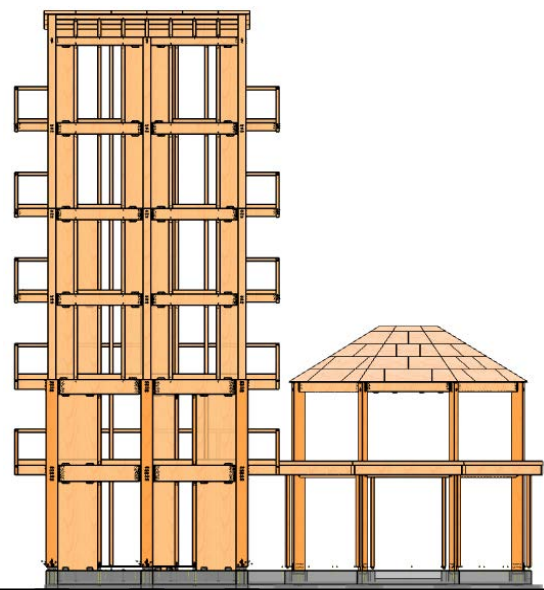
西立面図
