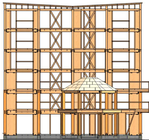
南立面図
