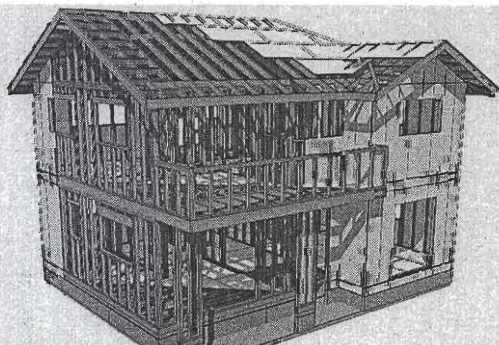
2×4CADパース図
